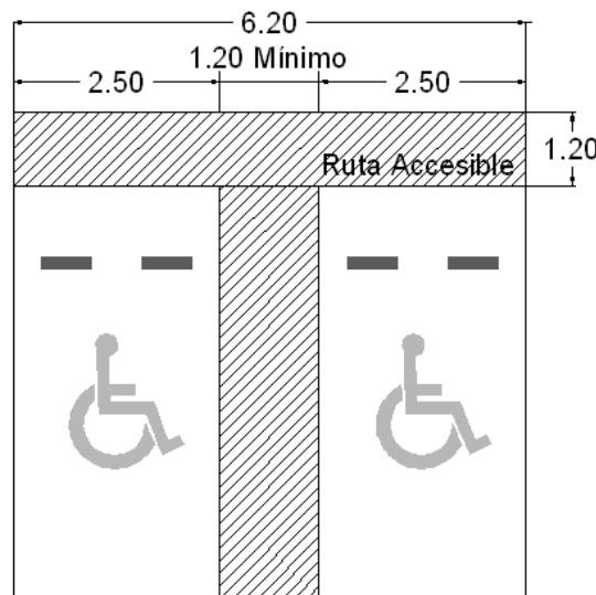
PLANTA ARQUITECTONICA
