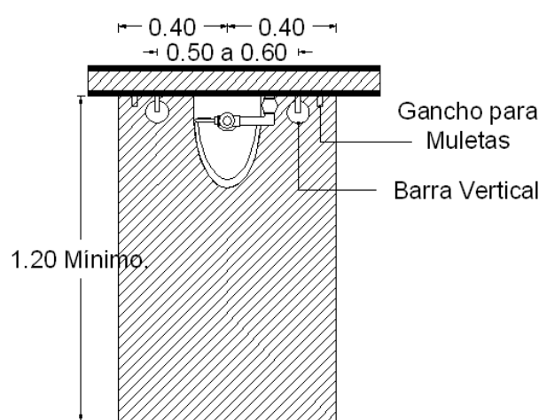
PLANTA ARQUITECTONICA
