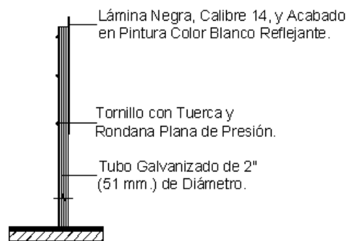
VISTA LATERAL
