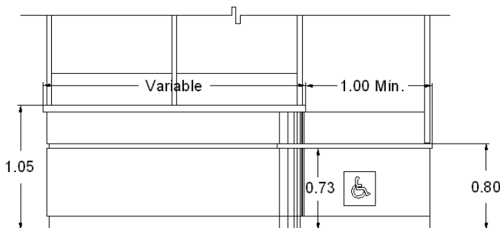
ALZADO FRONTAL
