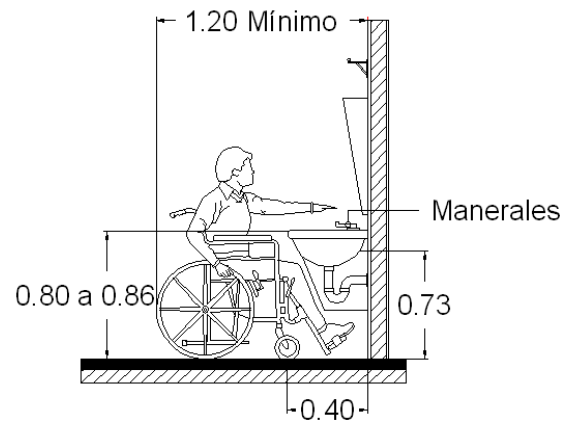
ALZADO LATERAL
