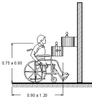
ALZADO LATERAL
