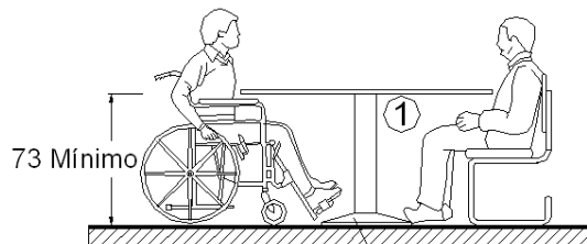
ALZADO LATERAL
