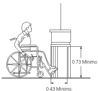
ALZADO LATERAL
